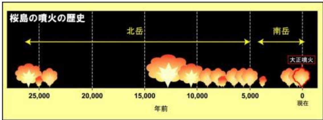
図 14 桜島の大規模噴火の歴史
