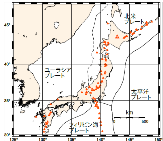
図 13 日本周辺のプレート境界と活火山の分布。
