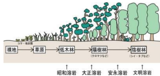
図 15 桜島の各時代に噴出した溶岩に繁茂する植生の時間経過による遷移
