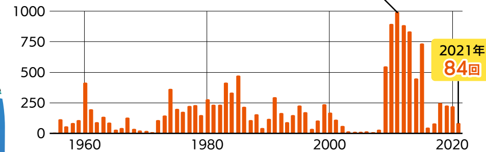
桜島の爆発回数
