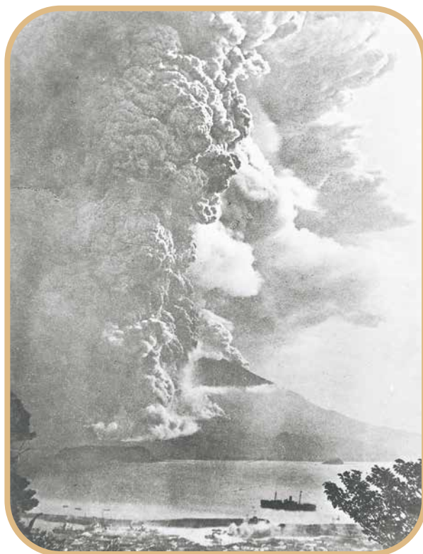
大正噴火のようす
