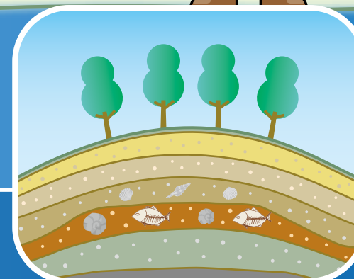
長い年月をかけ、大地がおし上げられ陸上で地層が見られるようになる
