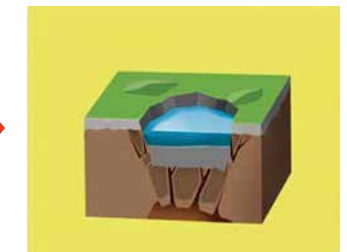
海水が入ってきて、錦江湾(湾奥部)が誕生しました。
