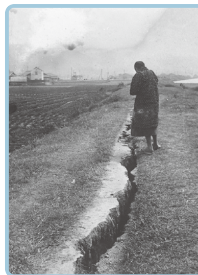
桜島地震による地割れ
