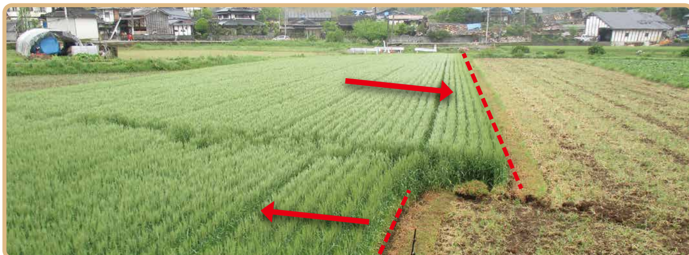
地表にあらわれた大地のずれ(断層)
