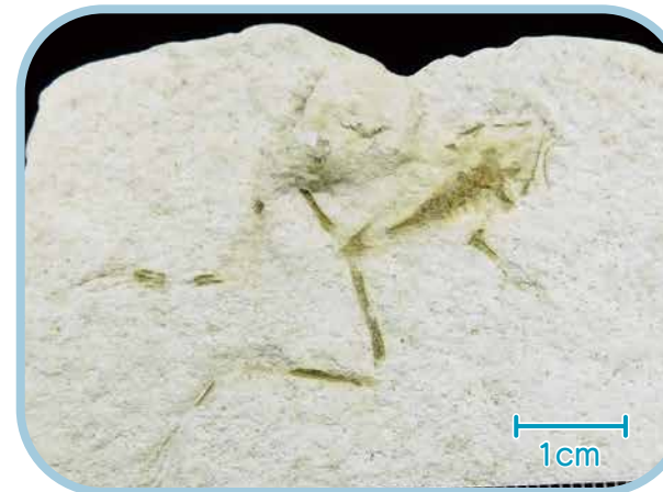
カエルの化石 (薩摩川内市)
