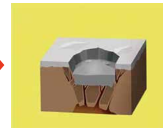
地下が空っぽになり、地面が落ちたことで大きな穴(カルデラ)ができました。
