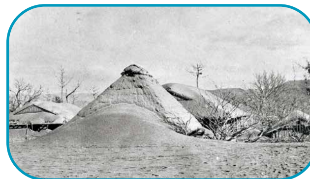
大正噴火の火山灰でうもれた家
